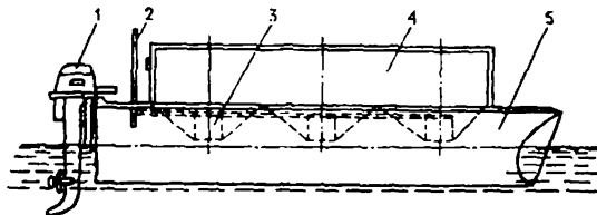
Рис. 8. Кормораздатчик СКР-1,5:
