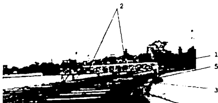
Рис. 18. Линия для раздачи кормов в рыбоводных садках: 1 — эстакада; 2 — бункер; 3 — кормораздатчики; 4 — бункер; 5 — дозатор; 6 — кормушка; 7 — поплавок; 8 — садки
