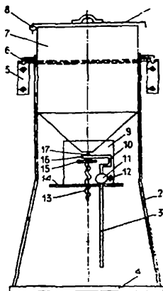
Рис. 12. Одномаятниковая кормушка Рефлекс-Т: 1 — крышка бункера; 2 — стойка поддона; 3 — маятник; 4 — поддон; 5 — крошштейн; 6 — крючья; 7 — бункер; 8 — петля крышки; 9 — защитный кожух; 10 — изгиб маятника; 11 — паровая опора; 12 — стопорный винт; 13 — стойка с винтовой нарезкой; 14 — поперечная планка; 15 — диск; 16 — кольцевой сбрасыватель; 17 — штырь
