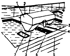
Рис. 19. Устройство для раздачи корма в садках: 1 — двухсекционный бункер; 2 — крыша; 3 — разгрузочный дозатор; 4 — стойка; 5 — обслуживающая площадка; 6 — кормовой столик
