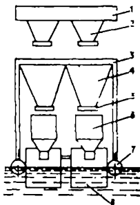
Рис. 18. Линия для раздачи кормов в рыбоводных садках: 1 — эстакада; 2 — бункер; 3 — кормораздатчики; 4 — бункер; 5 — дозатор; 6 — кормушка; 7 — поплавок; 8 — садки
