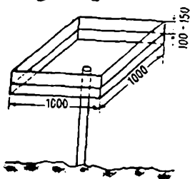
Рис. 15. Деревянный кормовой столик
